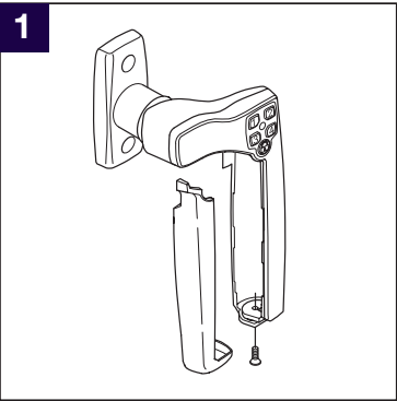
1. Använd medföljande torxnyckel och lossa skruven i änden på handtaget. Tag bort batteriluckan genom att skjuta den nedåt och vik ut. Tag ur de två batterierna.
